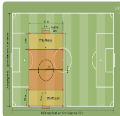
Kleinspielfeld für zwei tragbare Tore 5 x 2 m
